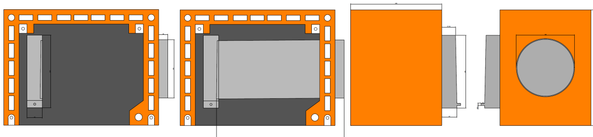
Bild 3 Schnittzeichnung Lüftungsstein (Darstellungen des Auftraggebers)
